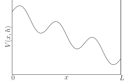
FIGURE 1.1 – Potentiel incliné par une force non-conservative.
