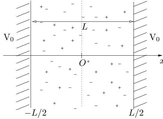
FIGURE 6.2 – Un électrolyte monovalent entre deux plans infinis séparés d’une distance L .
