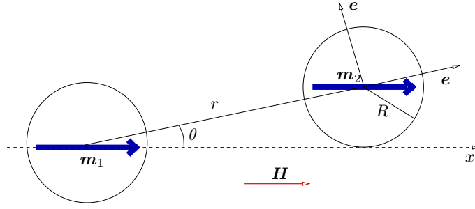
FIGURE 6.1 – Deux colloïdes magnétiques de moments magnétiques \mathbf{m}_1 et \mathbf{m}_2 séparés d’une distance r et plongés dans un champ d’excitation magnétique extérieur uniforme \mathbf{H} . L’angle \theta représente l’angle entre le rayon vecteur et le champ magnétique.
