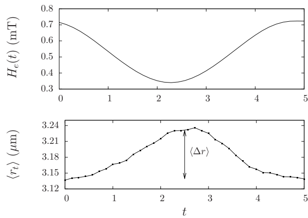
FIGURE 6.5 – Champ magnétique appliqué sur le doublet de colloïdes (en haut) et distance moyenne entre les particules mesurées expérimentalement (en bas) et tracés en fonction du temps.
